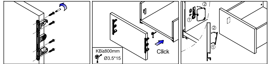
Montaje de la parte frontal
