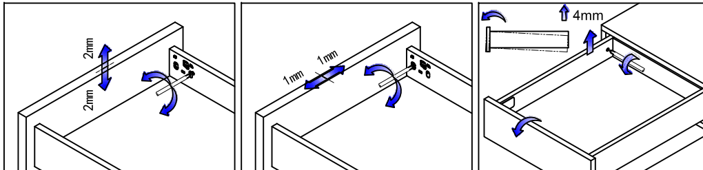
Ajuste de posición derecha/izquierda
