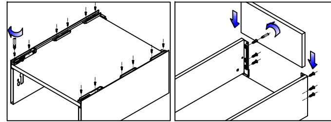
Montaje de la base
