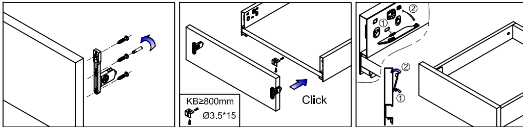
Montaje de la parte frontal
